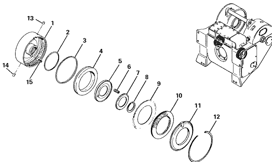
CLUTCH—NO. 44860
